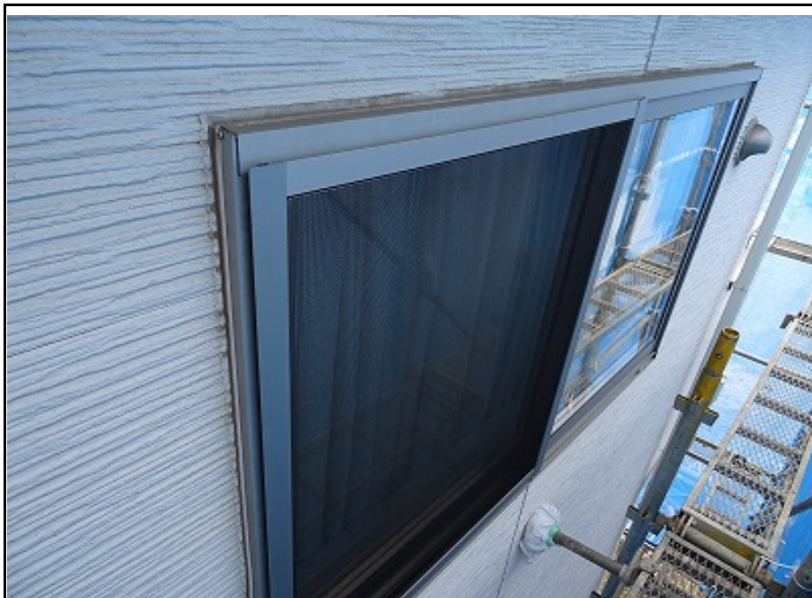
壁目地打ち替え (施工前)
