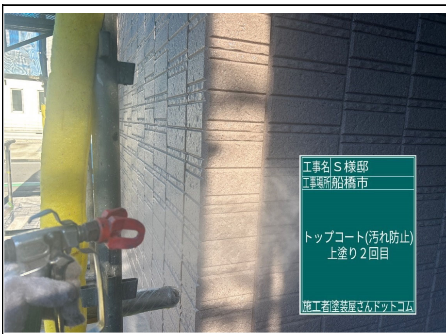
外壁 (トップコート上塗り2回目)
